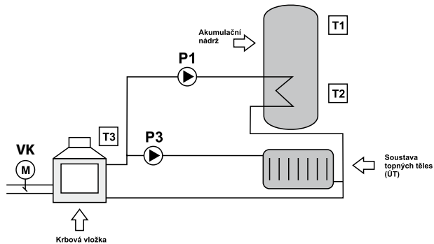
Základní provozní schéma regulátoru
