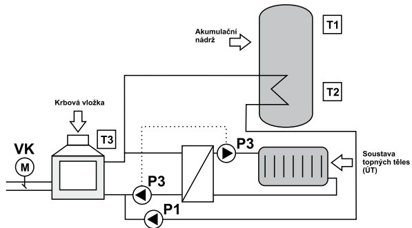
Provozní schéma regulátoru s výměníkem pro okruh ÚT (čerpadlo výměníku a připojeno k výstupu)
